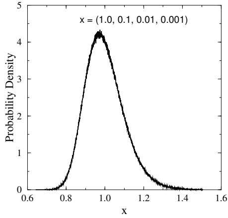
FIG. 3.14. PDF of the PC variable x(1.0, 0.1, 0.01, 0.001)
